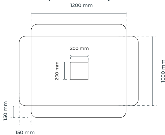
Tapa para IBC Modelo JRA (Sin calefacción)
