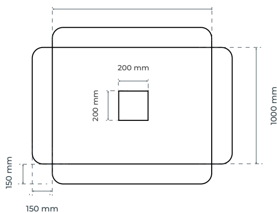
Tapa para IBC Modelo JRA (Sin calefacción) 1200 mm
