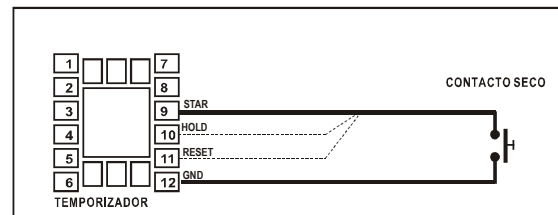
Figura 04 - Conectando contacto seco (relé, interruptor)
