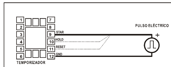
Figura 03 - Conectando un sensor tipo Pulso Eléctrico
