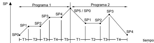
Fig. 11 - Ejemplo de programa 1 e 2 "linkados" (interconectados)
