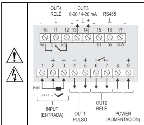
Figura 1 – Conexiones eléctricas
