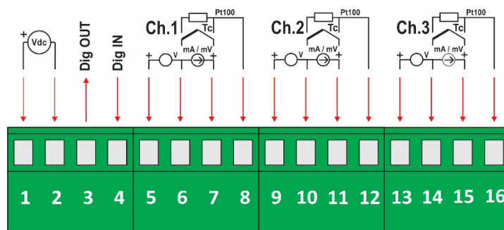
Figura 50 – Conexiones eléctricas
