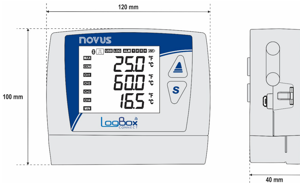
Figura 48 – Dimensiones de LogBox BLE
