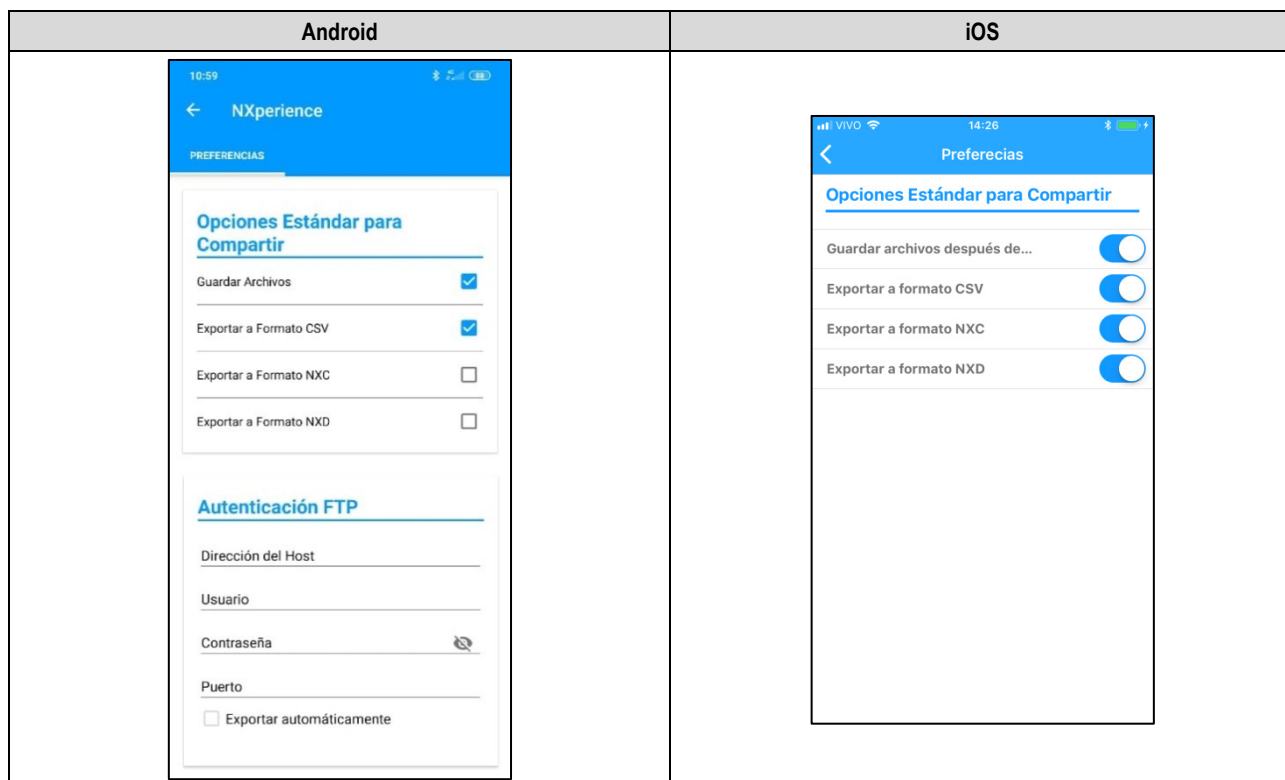
Figura 42 – Pantalla de preferencias
