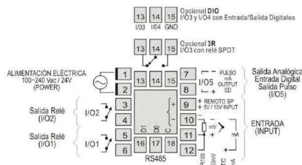
Figura 1 - Conexiones del panel trasero
