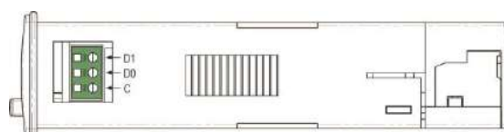
Fig. 03 – Conexiones de la comunicación serial RS485
