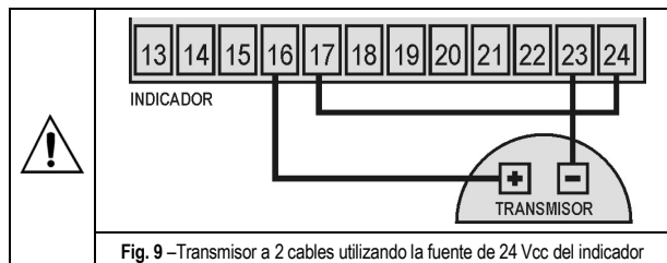
Fig. 9 – Transmisor a 2 cables utilizando la fuente de 24 Vcc del indicador
