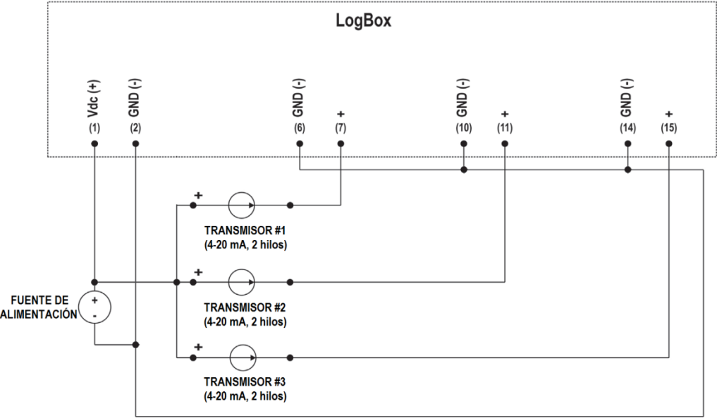
Figura 52 – Ejemplo de conexión de transmisores alimentados por el loop
