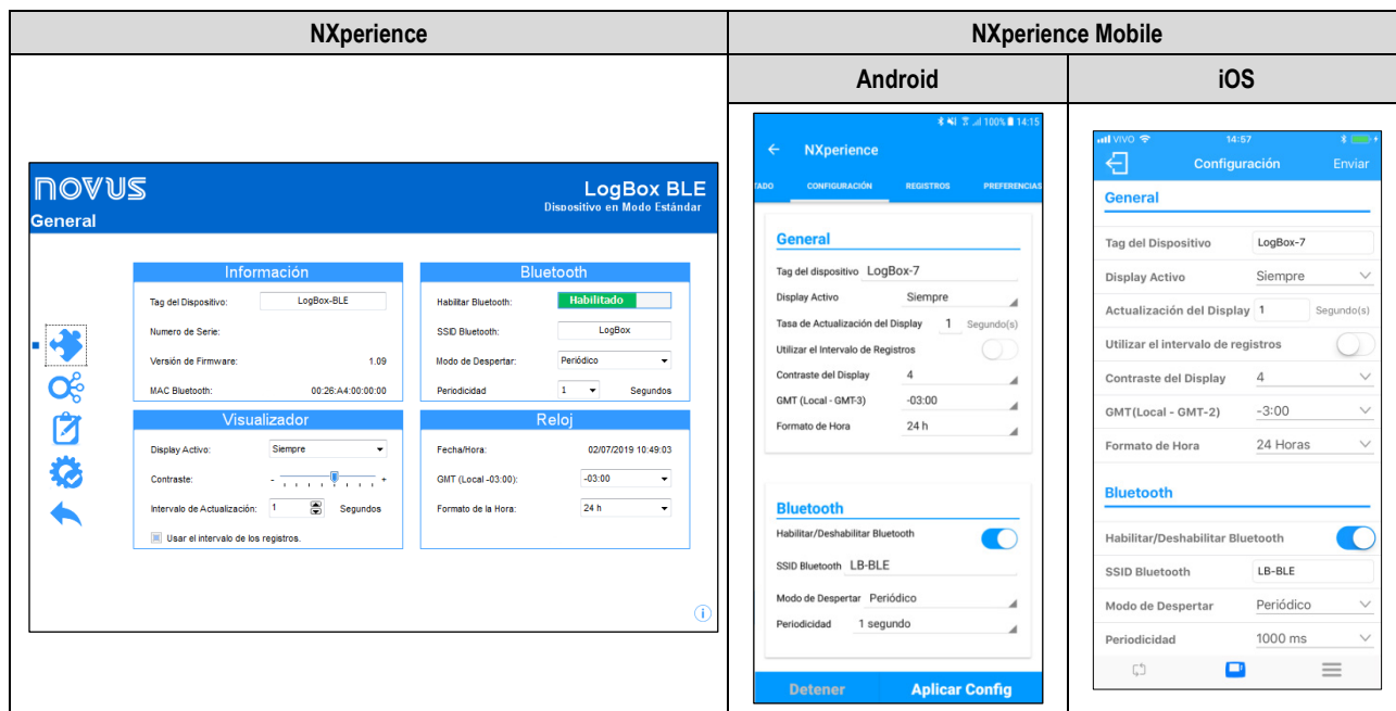
Figura 3 – Parámetros Generales
